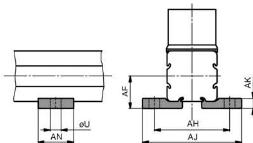
OSP-P16至P80系列: E1型 (使用1个螺钉从上/下安装)
