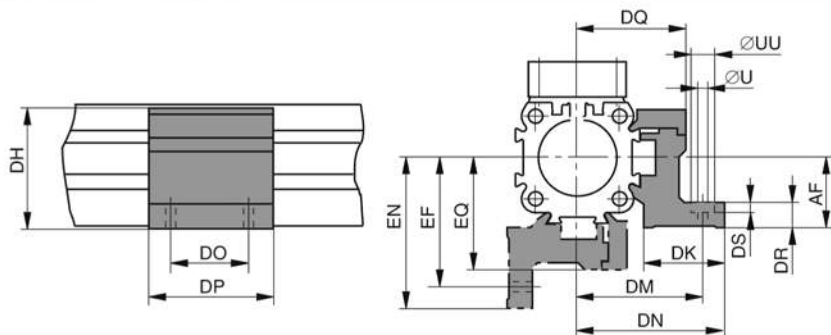
OSP-P16至P80系列: D1型 (使用2个螺钉从下安装)
