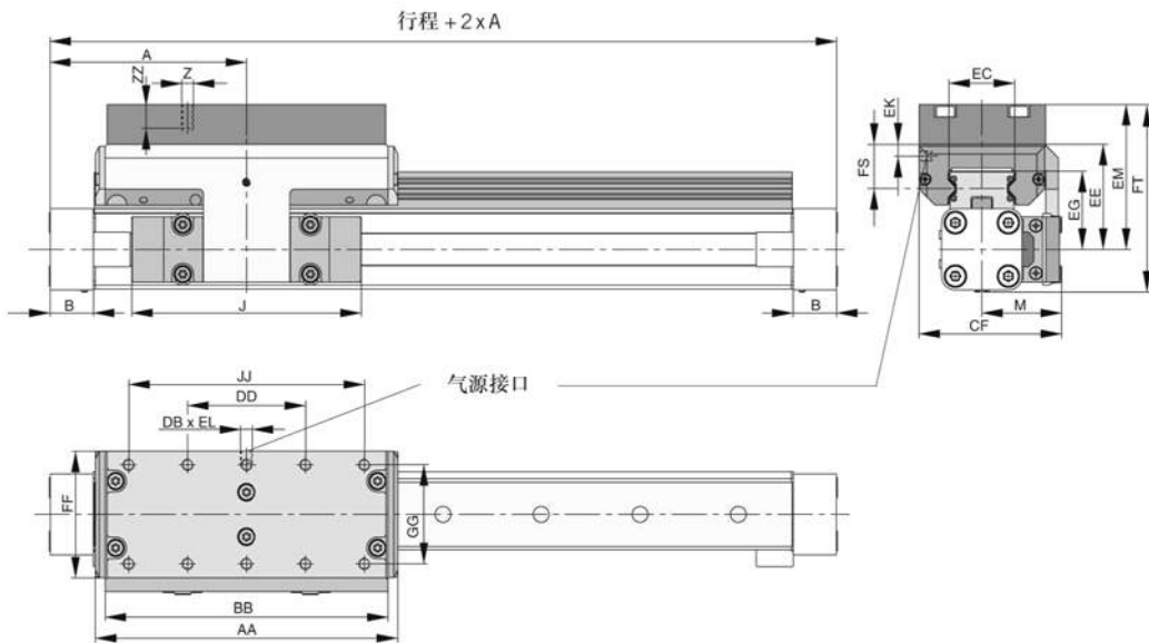
尺寸表 (mm) OSP-P MB-PL25, MB-PL32, MB-PL40, MB-PL50系列
