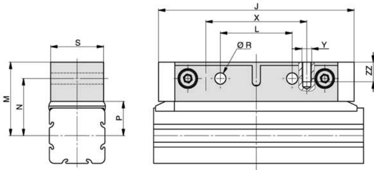
滑块 OSP-P10系统
