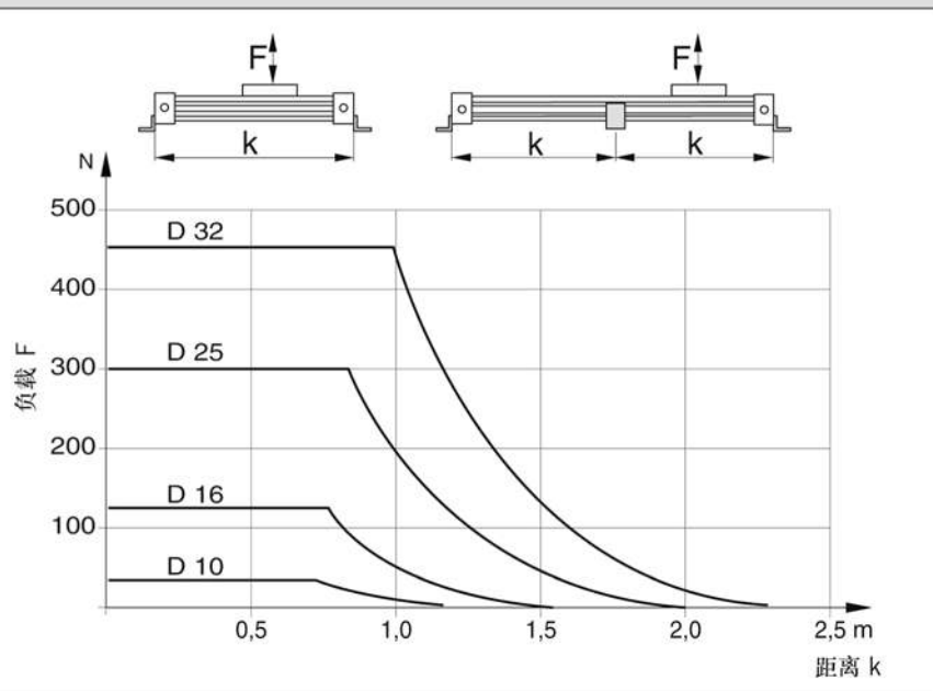
允许支撑间距：OSP-P10-P32
