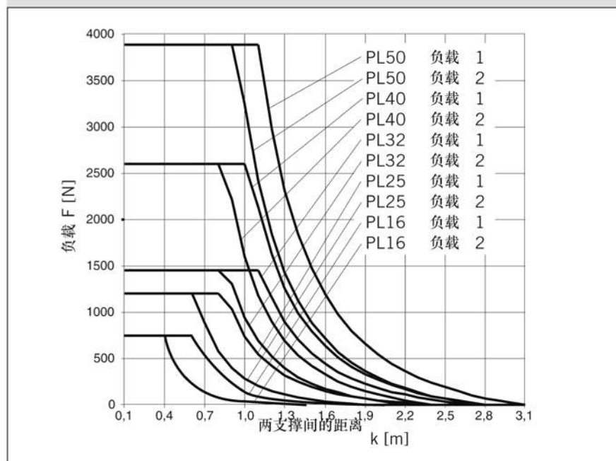
允许的无支撑长度 PL16, PL25, PL32, PL40 和 PL50
