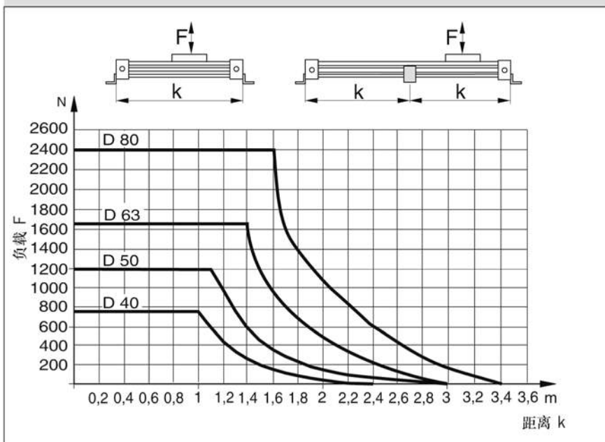
允许支撑间距：OSP-P40-P80
