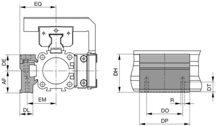
图纸说明: 带有STL导轨装配图。
