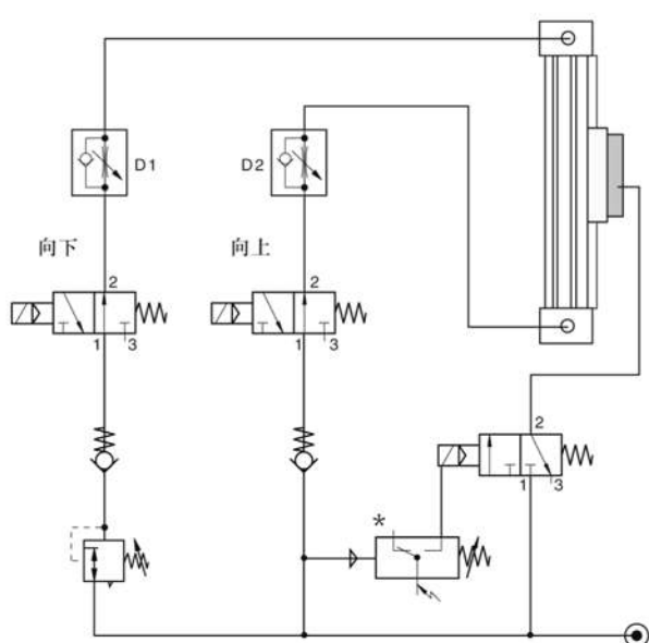
用3/2阀控制气缸。 基本位置-加压
