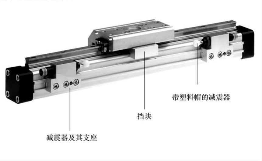
根据质量和速度来选择减震器 OSP-KF16系列
