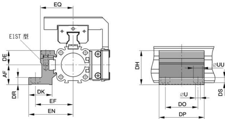
图纸说明: 带有STL导轨装配图。
