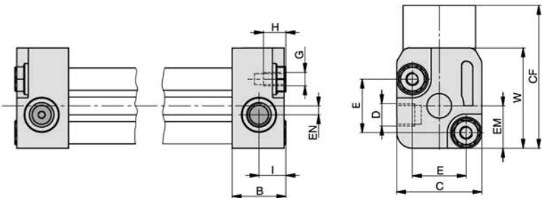
端盖/气源接口 OSP-P10系统
