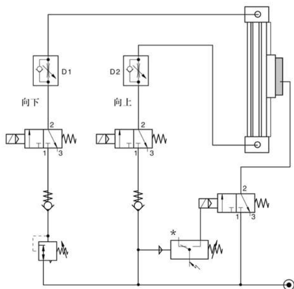
用3/2阀控制气缸。 基本位置-排气
