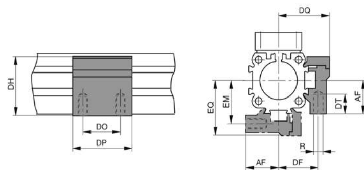
OSP-P16至P80系列: D1型 (使用2个螺钉从下安装)
